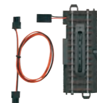
20997 Entkupplungsgleis - 94,2 mm. - Inhalt: 1 Stück. - Entkupplungsgleis zum manuellen und elektrischen Entkuppeln geeignet. Der elektrische Betrieb ist ausschließlich in Verbindung mit dem Stellpult 72752 und dem mitgelieferten Kabel möglich. € 31,99*
